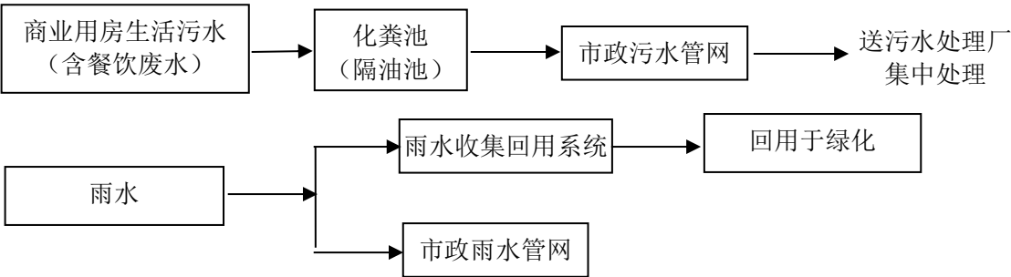
图 3-1-1 废水处理工艺
