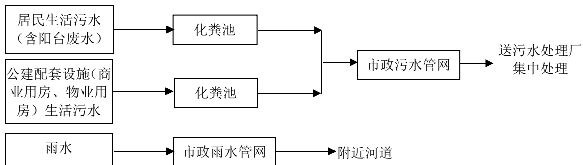
图 3-1-1 废水处理工艺
