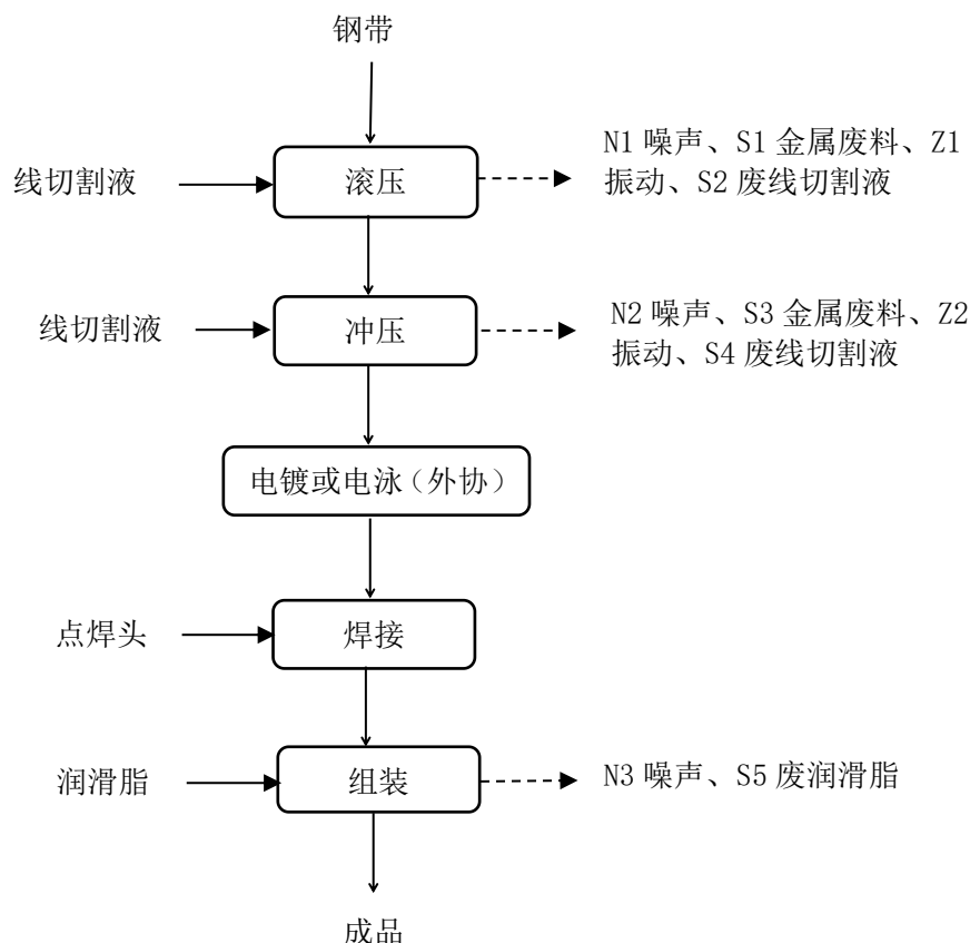
图 2-3-1 生产工艺流程图
