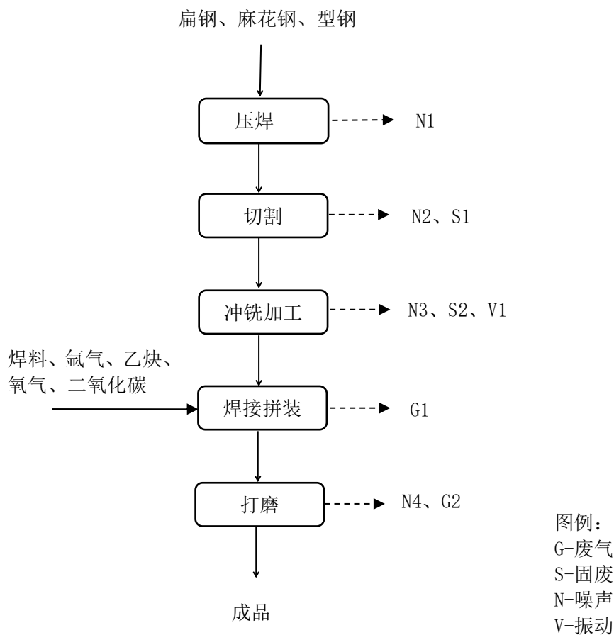
图 2-3-1 钢格板生产工艺流程图
