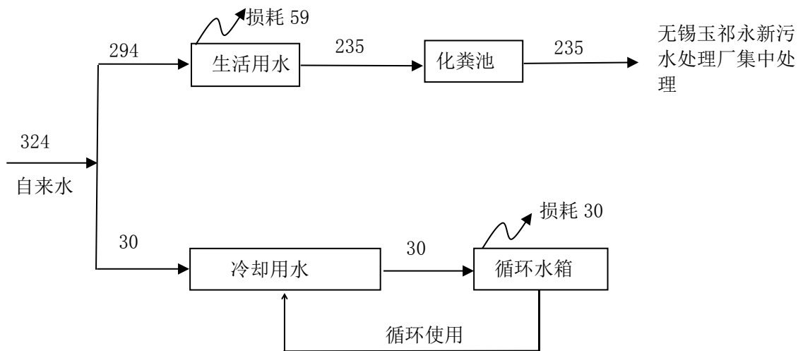
图 2-2-2 全厂实际水平衡图 单位 t/a
